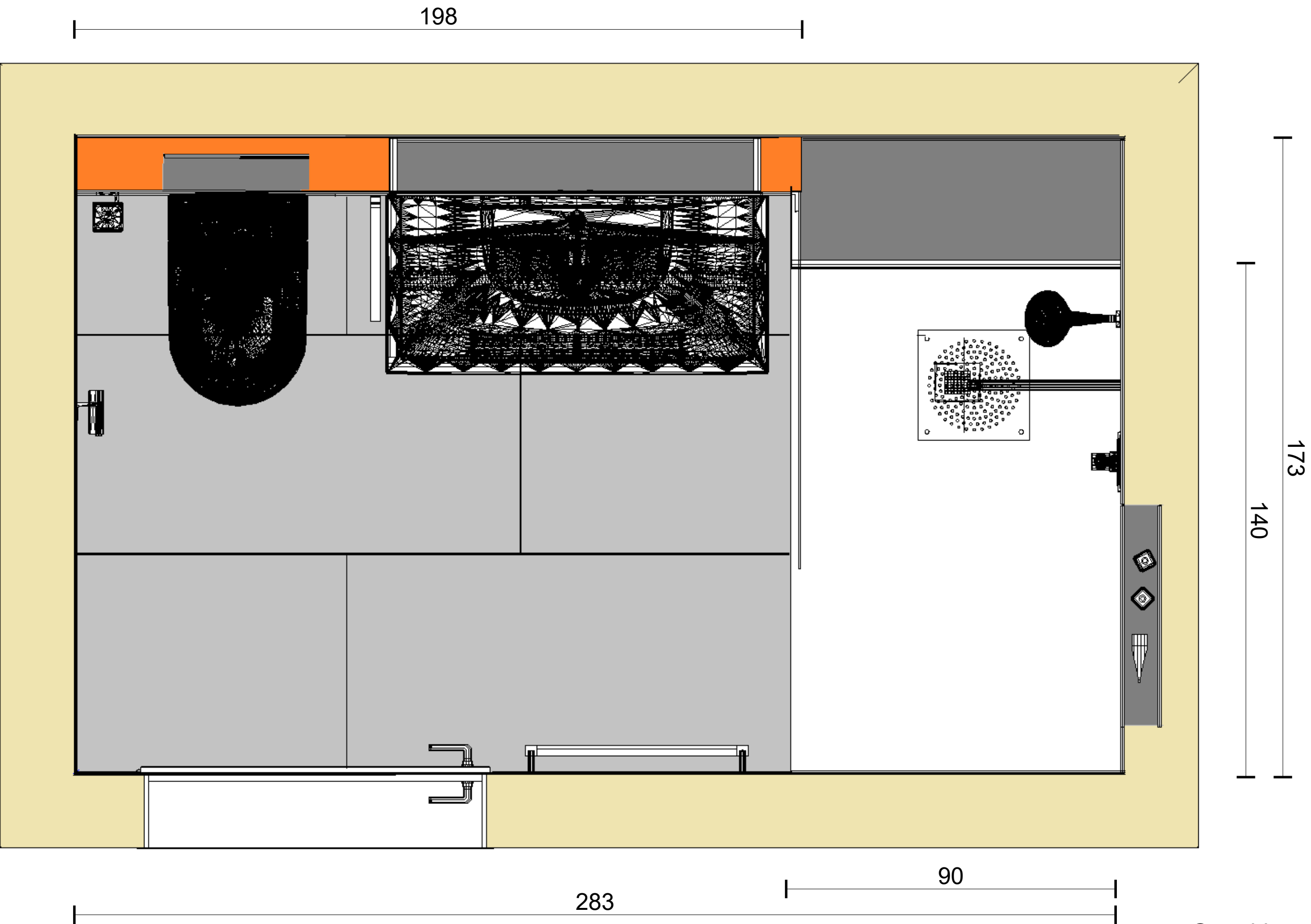
Grundriss
